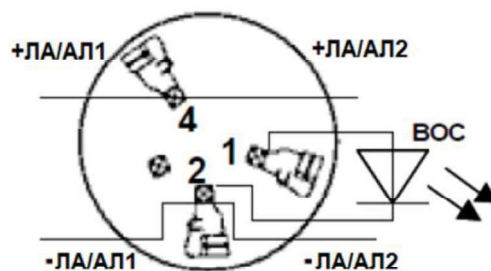
Рис. 1. Подключение базового основания SF-B1
